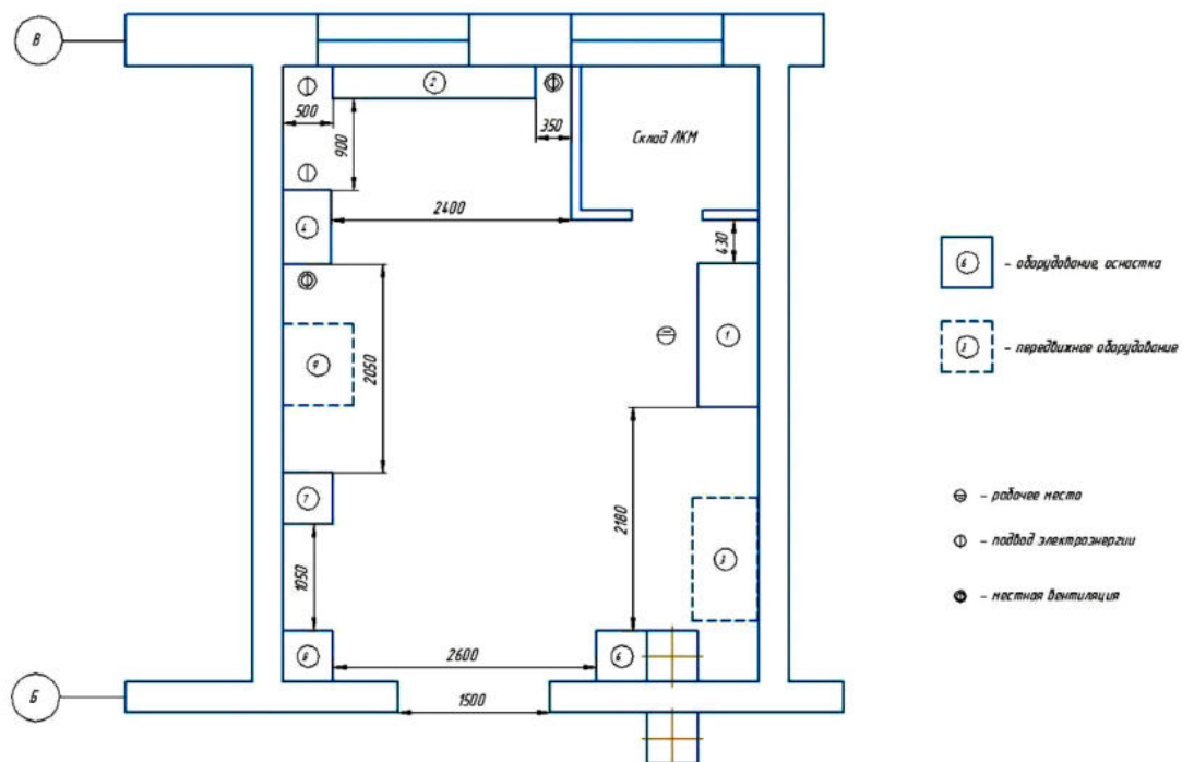
Рисунок 6. Планировка участка
