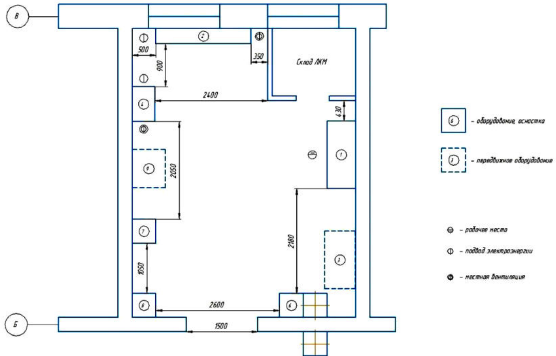
Рисунок 6. Планировка участка
