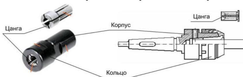
Рис.25 Сверлильный цанговый патрон
