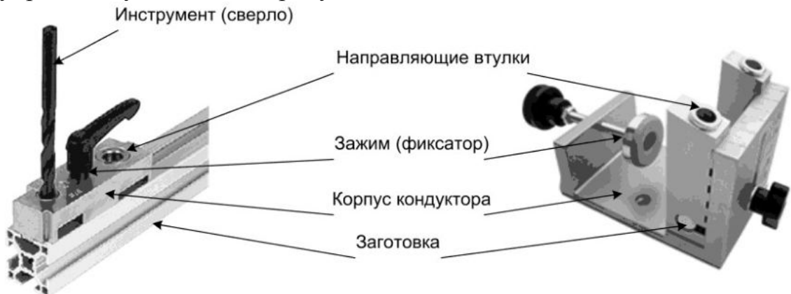
Рис.7 Кондуктор
