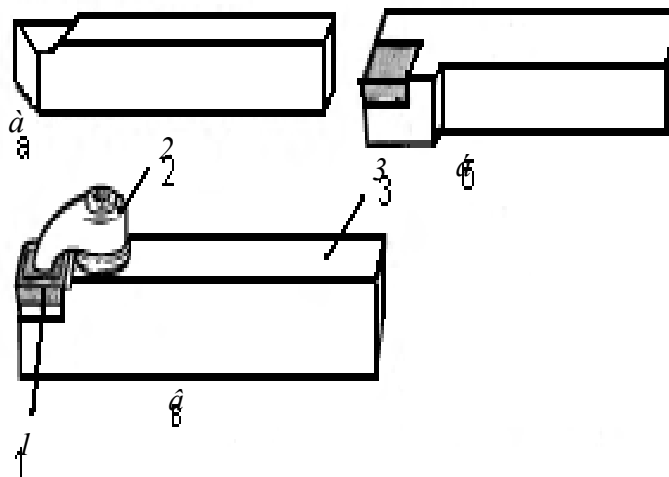
Рис. 10. Резцы:
