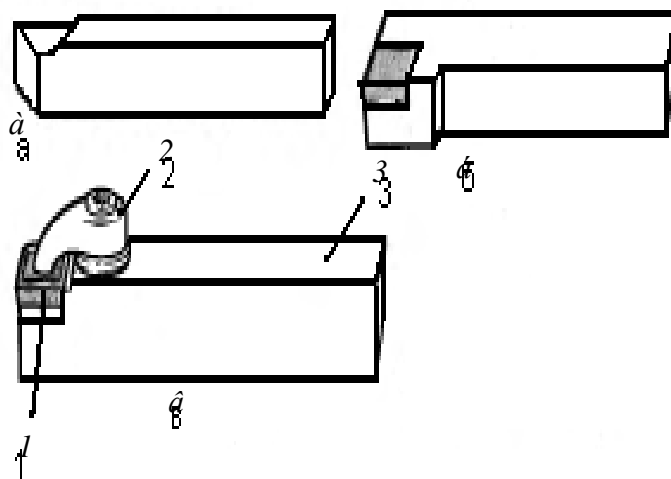
а — цельные; б — с припаянной пластинкой твердого сплава; в — с механическим креплением пластинки твердого сплава; 1 — режущая пластина; 2 — прихват; 3 — державка
