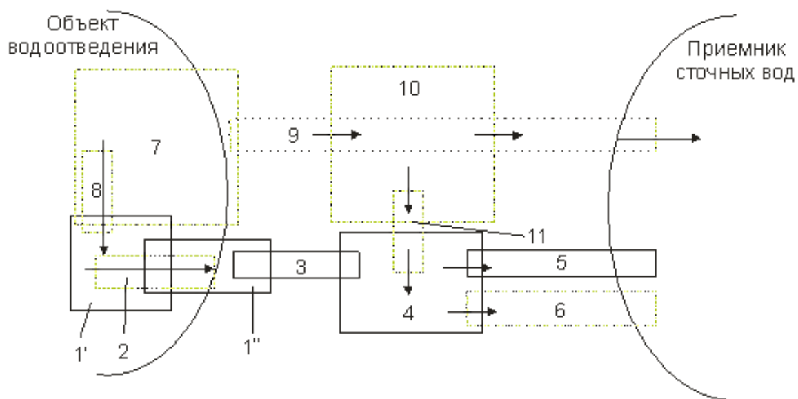
Рис.6. Блок-схема водоотведения.
