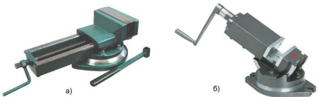
Рис.4 Тиски а) тиски машинные; б) тиски поворотные
