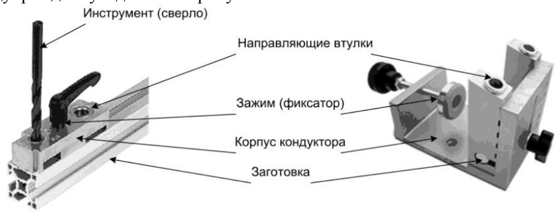
Рис.7 Кондуктор
