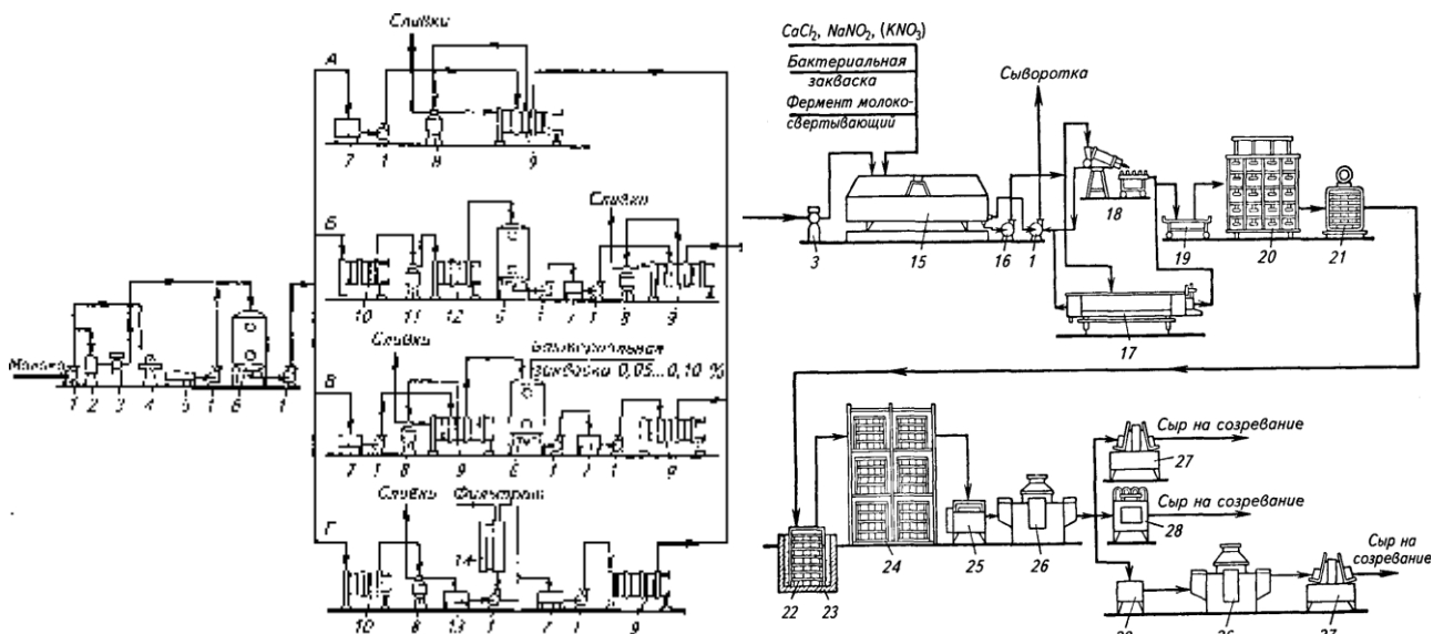
Рисунок.4. Типовая аппаратурно-технологическая схема производства сыров
