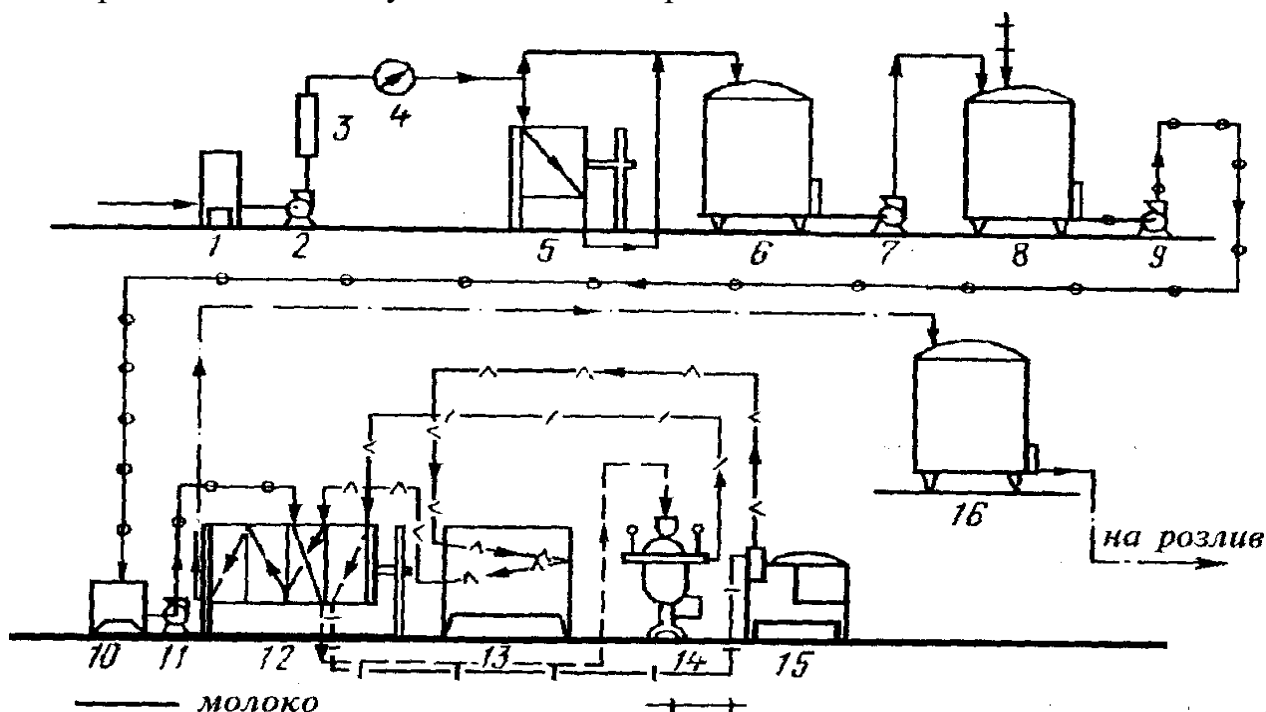
Рисунок 1. Аппаратурно-технологическая схема производства пастеризованного молока
