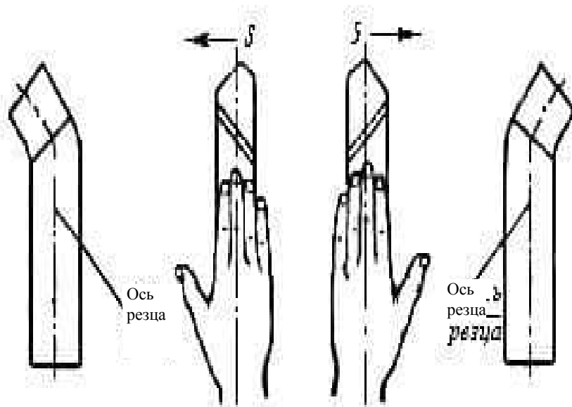
Рис. 9. Определение правого и левого резца:
