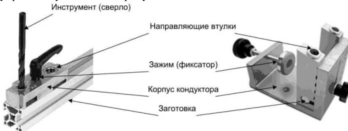
Рис.7 Кондуктор
