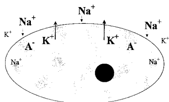
РАСПРЕДЕЛЕНИЕ ИОНОВ ПО ОБЕ СТОРОНЫ МЕМБРАНЫ КЛЕТКИ
