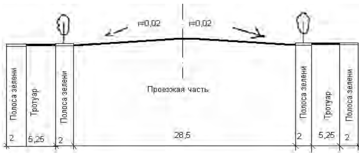
Рис. 10. Поперечный профиль улицы без полосы для разделения встречного движения.
