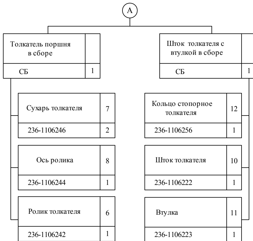
Рис. 6.7. Структурная схема разборки топливopодкачивающего насосa двигателя ЯМЗ-238Н
