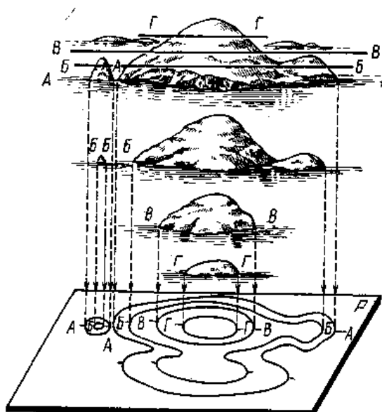
Рисунок 1 - Образование горизонталей
