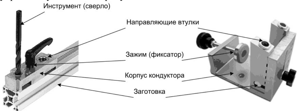
Рис.7 Кондуктор
