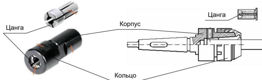
Рис.25 Сверлильный цанговый патрон
