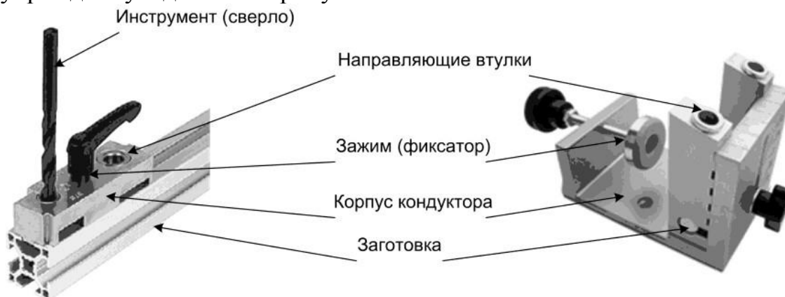
Рис.7 Кондуктор
