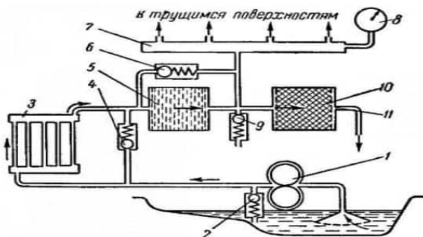
Рисунок 3.1.: Принципиальная схема системы смазки тракторного двигателя:
