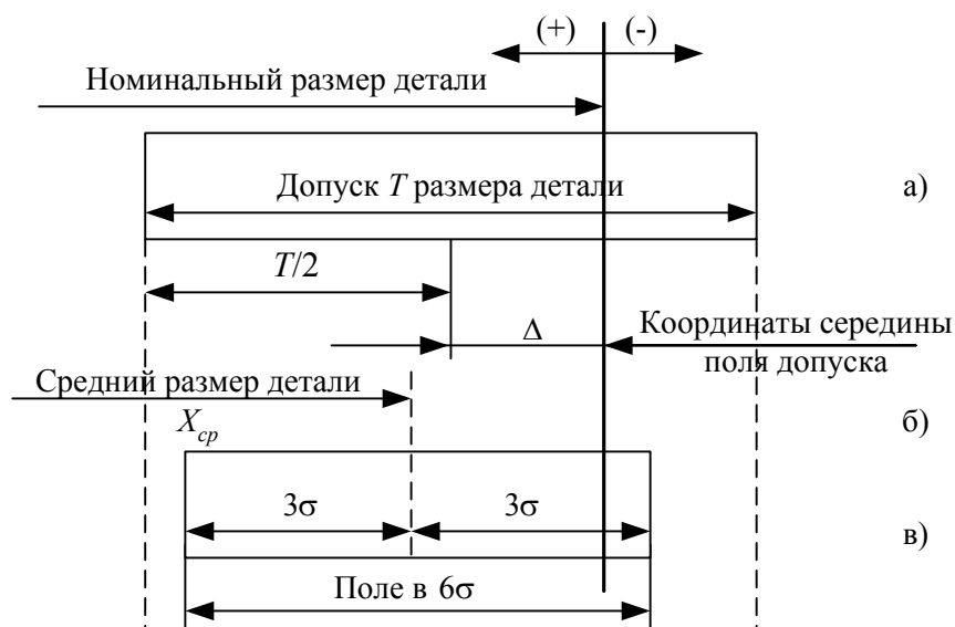
Рис. 6.18. Построение поля в 6\sigma
