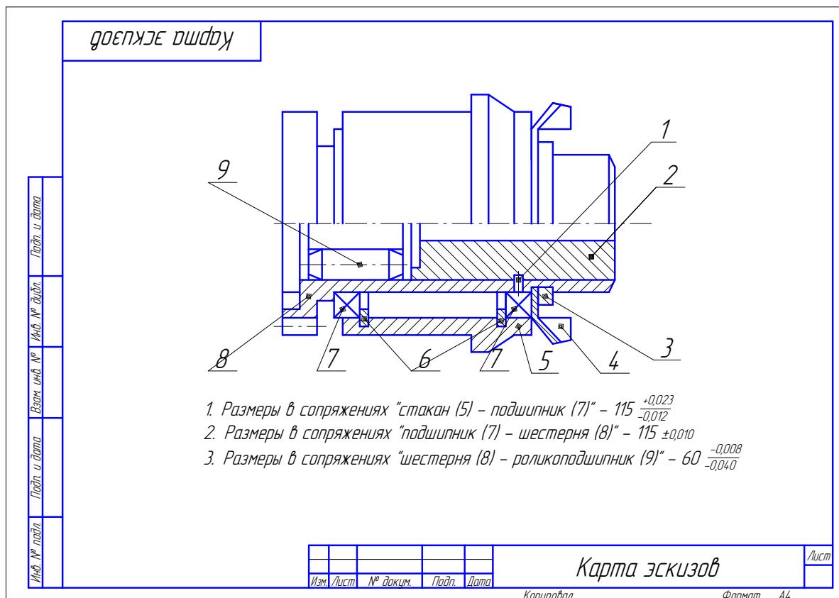
Рис. 6.15. Карта эскизов процесса сборки
