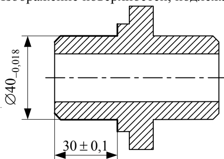
Рис. 6.10. Изображение поверхностей, подлежащих обработке.
