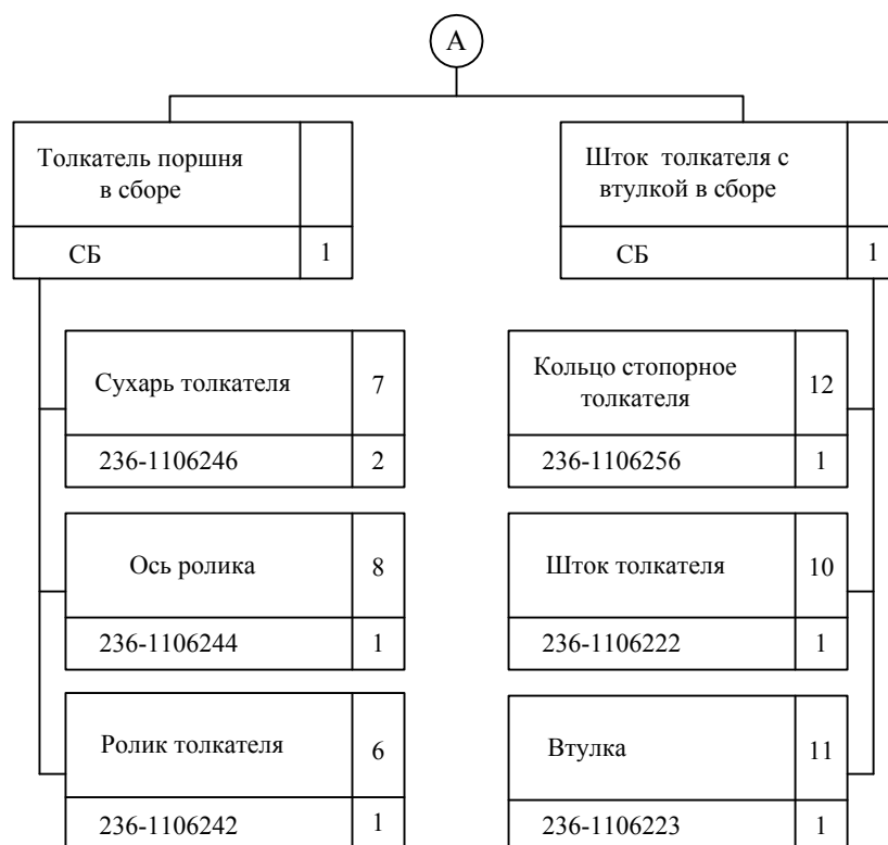
Рис. 6.7. Структурная схема разборки топливopодкачивающего насоса двигателя ЯМЗ-238Н
