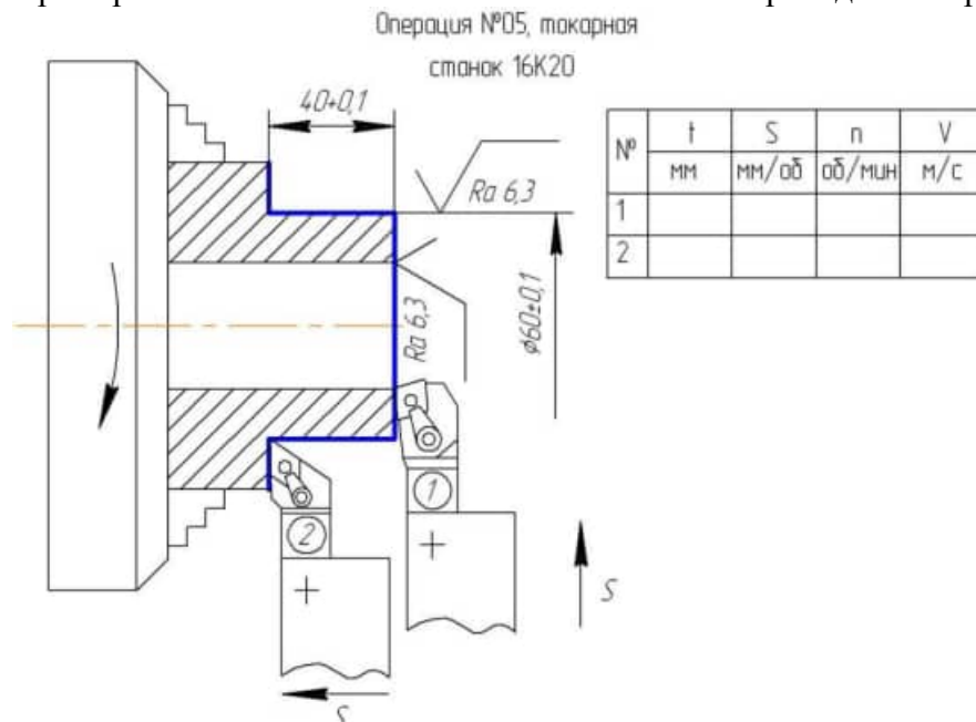
Рис. 1. Технологический эскиз операции 05 «Токарная»
