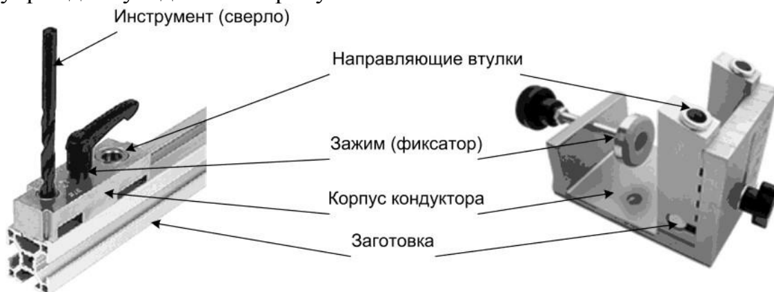
Рис.7 Кондуктор
