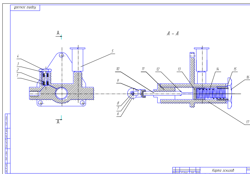
Рис. 6.8. Карта эскизов технологического процесса разборки топливopодкачивающего насосa двигателя ЯМЗ-238Н
